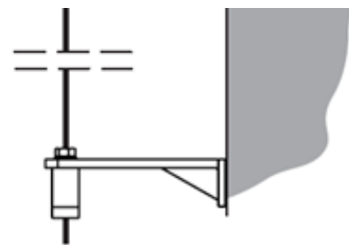
Support de montage avec tendeur de façade
