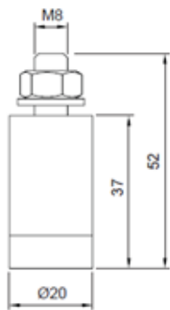
Tendeur de façade
